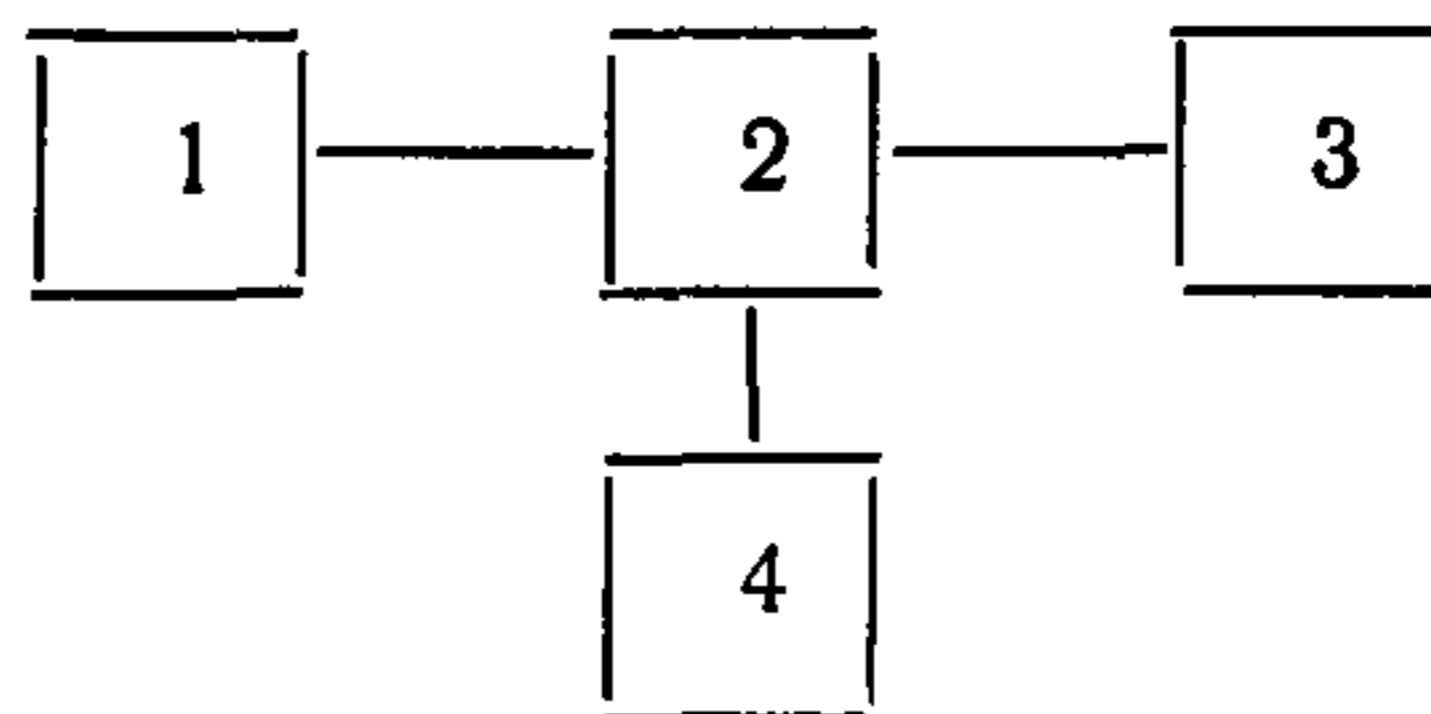
1—измерительный генератор; 2—коаксиальный соединитель; 3—поверяемый вольтметр; 4—образцовый частотомер
