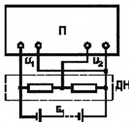
Рисунок 3 — Схема проверки делителя напряжения методом измерения входного и выходного напряжений
