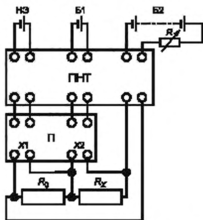
П — потенциометр постоянного тока; ПНТ — переключатель направления тока; R_0 — эталонная мера сопротивления; R_x — измеряемое сопротивление; R — регулировочный магазин сопротивлений; H3 — нормальный элемент; B1, B2 — источники питания; X1, X2 — зажимы потенциометра
