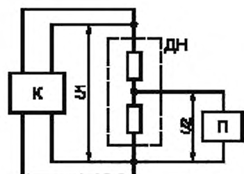
Схема измерения калибратором
