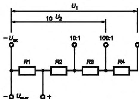
Рисунок 4 — Схема проверки делителя напряжения методом опорного напряжения, лист 1
