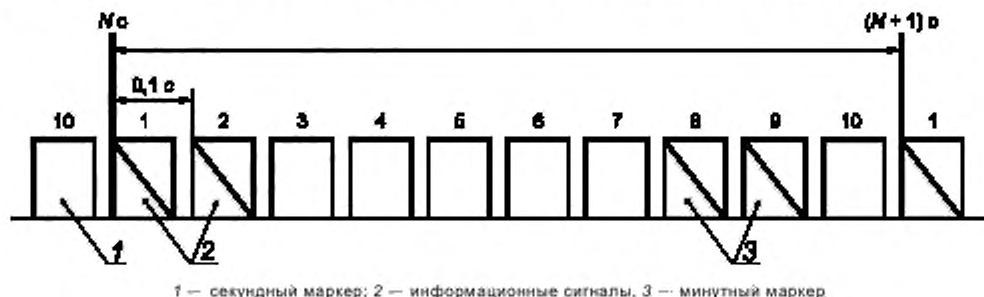
Рисунок 1 — Информационная структура сигнала
