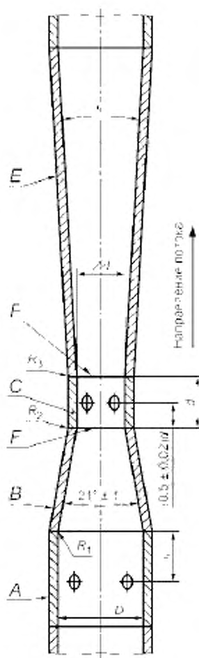
Е — диффузор; С — горловина; В — сужающаяся коническая часть; А — входной цилиндрический участок; F — плоскости соединения элементов трубы Вентури; d — см. 5.4.7
