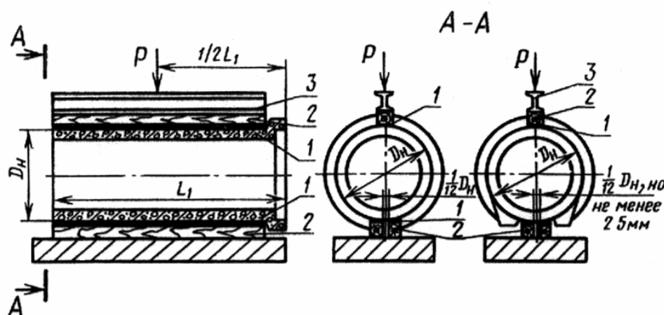
Схема испытания раструбной трубы
