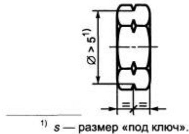
Рисунок 6 - Альтернативная маркировка левой резьбы
