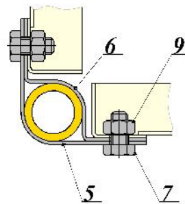
Рис. 2 Узел А
