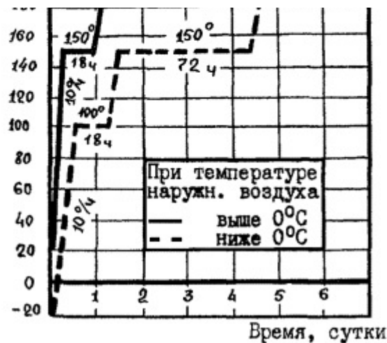
Рис. 7 Режим сушки и разогрева газоходов (из жаростойкого бетона на портландцементе с шамотным заполнителем), граничащих с грунтом
