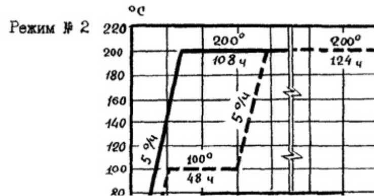
Рис. 1 Режим сушки и разогрева дымовых труб из жаростойкого бетона на портландцементе с шамотным заполнителем
