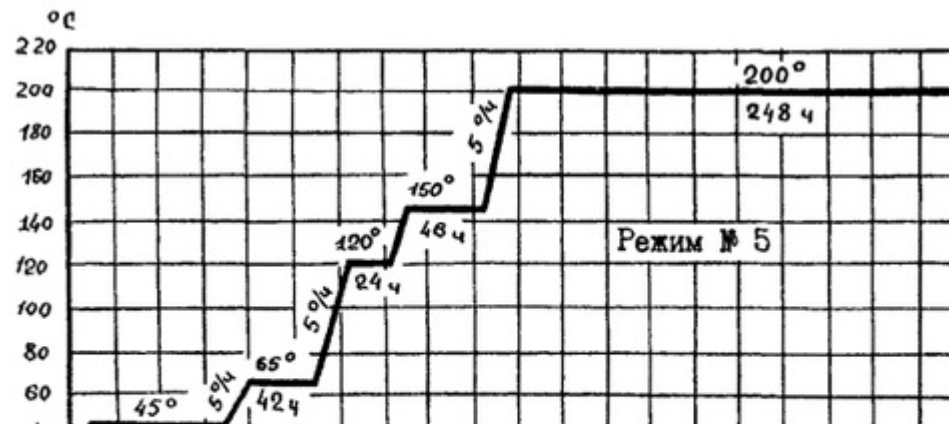
Рис. 4 Режим сушки монолитной футеровки железобетонных труб
