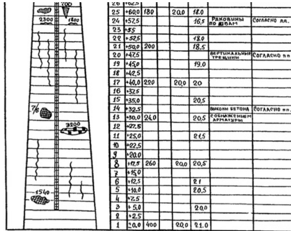
Условные обозначения дефектов и повреждений стволов железобетонных труб
