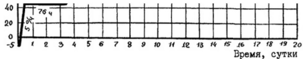
Рис. 5 Режим отогревания кирпичной кладки дымовой трубы (без футеровки) и газоходов, возведенных способом замораживания
