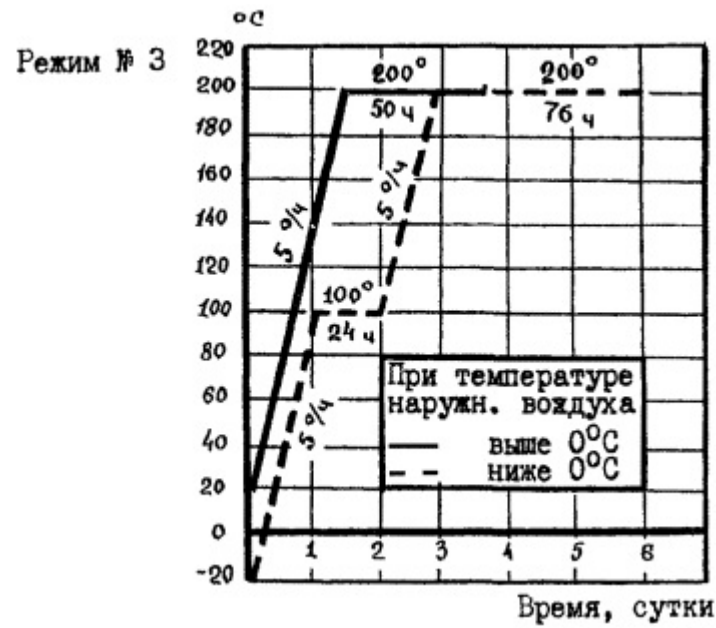
Рис. 3 Режим сушки футеровки кирпичных, железобетонных и стальных дымовых труб
