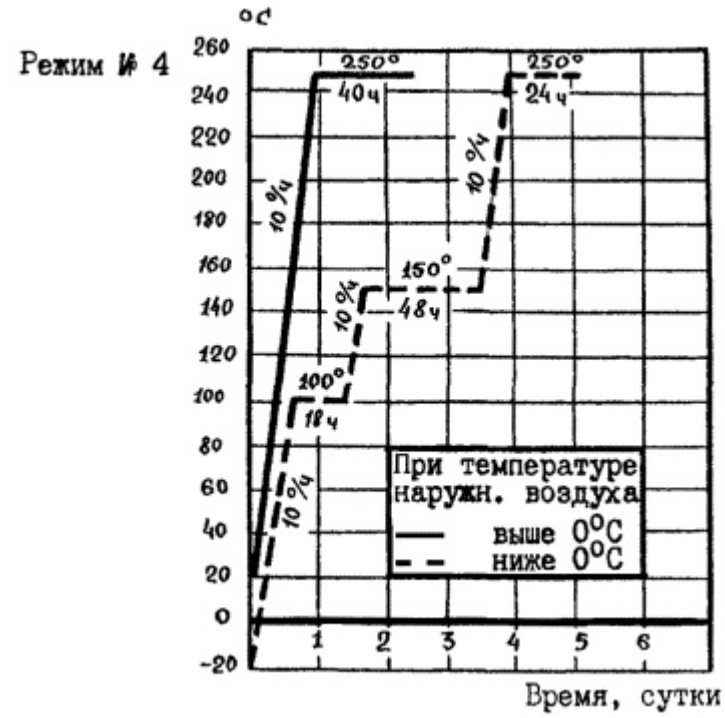
Рис. 4 Режим сушки монолитной футеровки железобетонных труб
