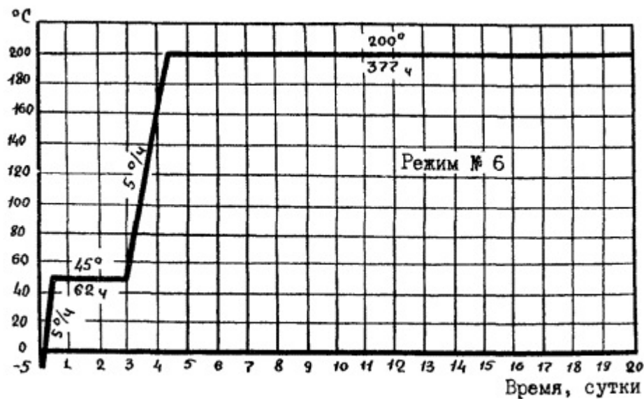
Рис. 6 Режим отогревания кирпичных дымовых труб с футеровкой (с теплоизоляцией или воздушным зазором), возведенных способом замораживания
