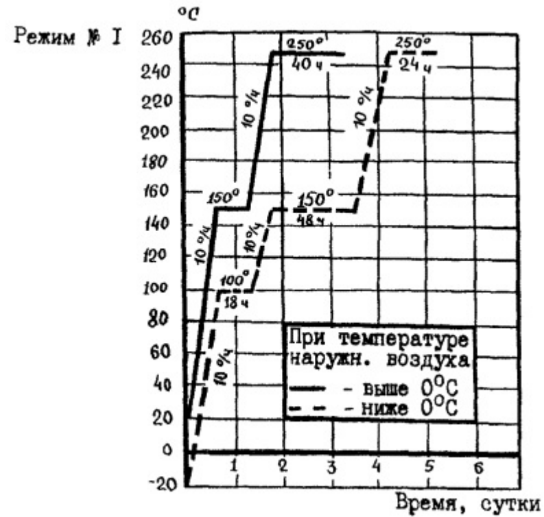
Рис. 1 Режим сушки и разогрева дымовых труб из жаростойкого бетона на портландцементе с шамотным заполнителем
