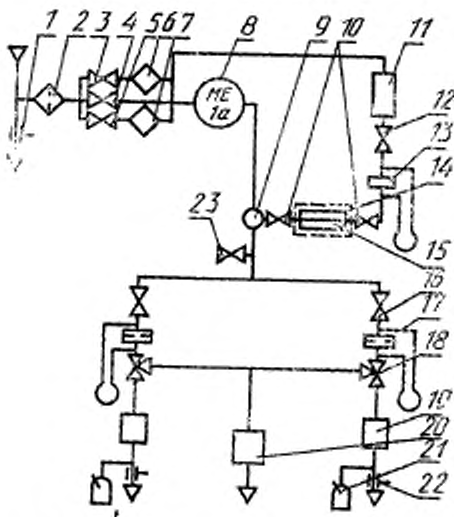
Схема динамической установки
