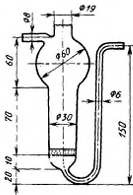
Склянка с фильтром для отбора пробы
