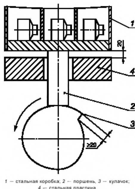
Рисунок 1 — Установка для механического воздействия
