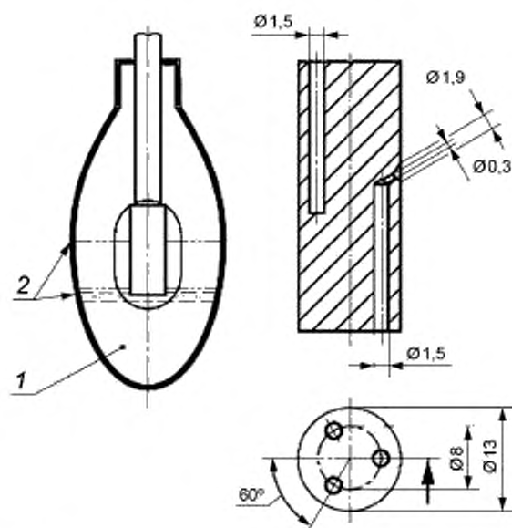
Рисунок 8 — Распылитель
