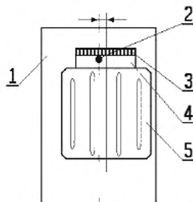
1 – щит; 2 – штырь; 3 – горизонтальная линейка; 4 – приспособление; 5 – ИДА
