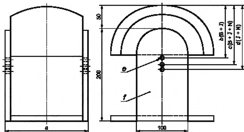
Рисунок А.2 — Макет головы В, J или N — по размерам выше базовой плоскости и измененный по ширине
