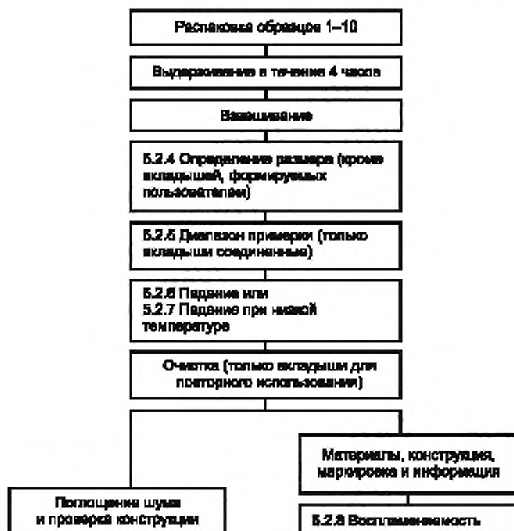
Рисунок В.3 — Блок-схема испытания вкладышей
