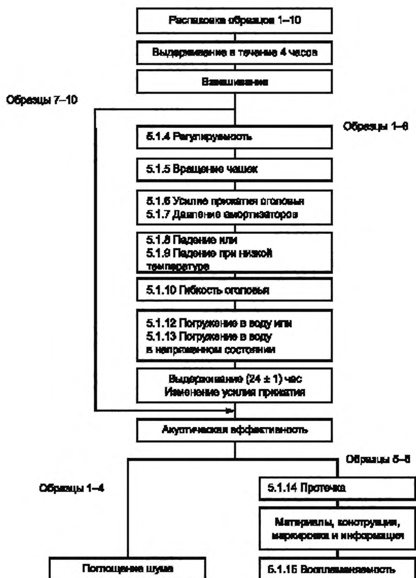
Рисунок В.1 — Блок-схема испытаний наушников с оголовьем
