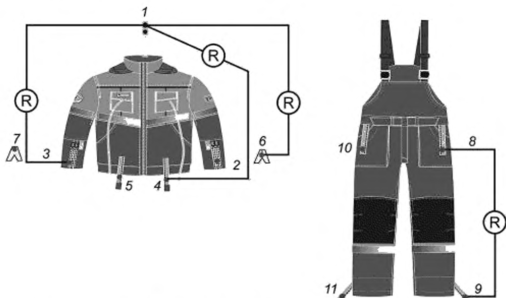
1 — контактный вывод на касника; 2, 3 — контактные выводы правого и левого рукавов; 4, 5 — контактные выводы от куртки к полукombineзону; 6, 7 — контактные выводы левого и правого зажимов переноса потенциала; 8, 10 — контактные выводы от полукombineзона к куртке; 9, 11 — контактные выводы от полукombineзона к ботинкам
