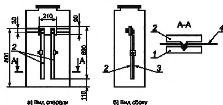
Рисунок 6 — Держатель испытуемого образца в испытательной камере
