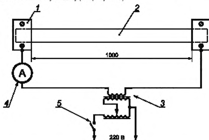
1 — разборные двоянные медные пластины; 2 — испытуемый образец; 3 — регулируемый источник напряжения; 4 — амперметр; 5 — выключатель
