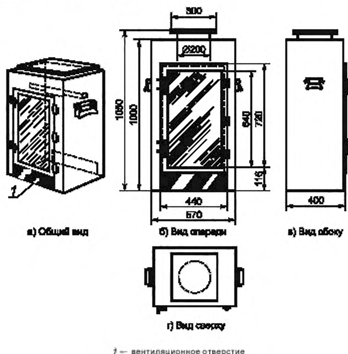
Рисунок 5 — Испытательная камера
