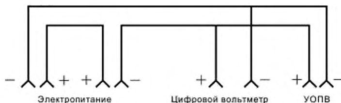
Рисунок 2 — Схема подключения цифрового вольтметра
