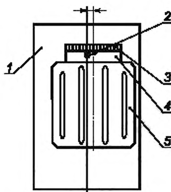
1 — щит; 2 — штырь; 3 — горизонтальная линейка; 4 — приспособление; 5 — ИФА
