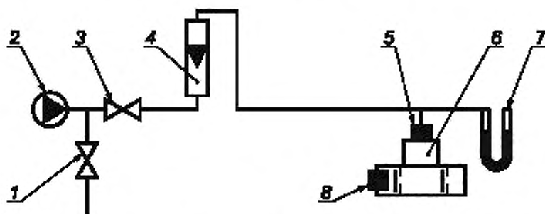
1, 3 — регулирующие вентили; 2 — устройство подачи воздуха; 4 — расходомер с верхним пределом измерения 0,063 м 3 /ч и приведенной погрешностью не более \pm 2,5\% ; 5 — присоединительное устройство; 6 — клапанная коробка; 7 — мановакуумметр с пределом измерения до 2500 Па и абсолютной погрешностью не более \pm 20 Па; 8 — пробка
