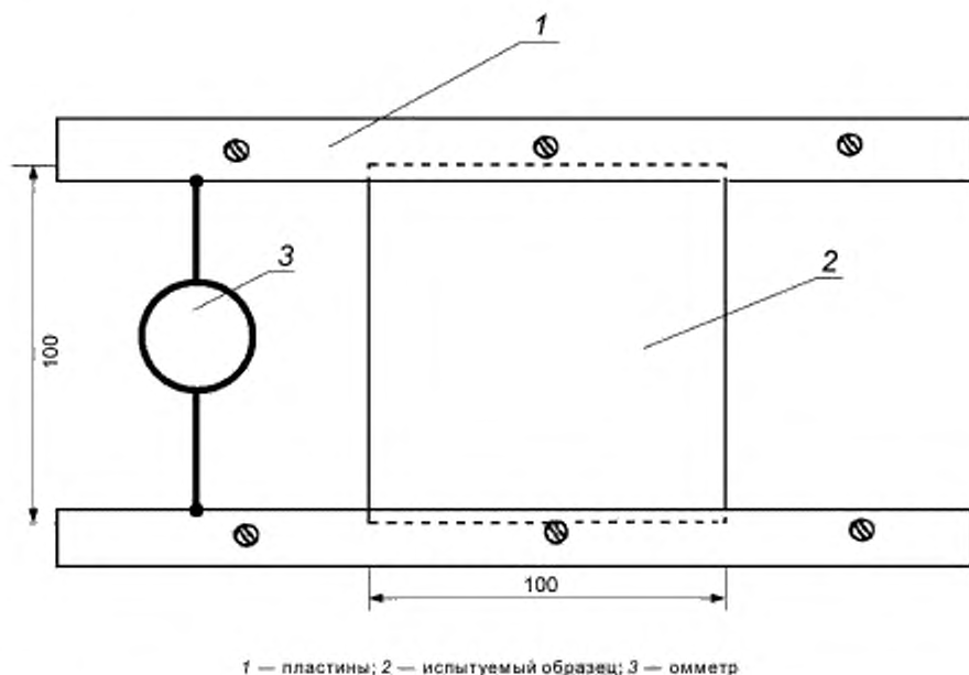
Рисунок 10 — Измерение электрического поверхностного сопротивления электропроводящей ткани
