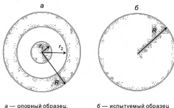
r_1 — радиус внутреннего проводника коаксиальной антенны, r_2 — внутренний радиус внешнего проводника коаксиальной антенны; R — радиус фланца коаксиальной антенны
