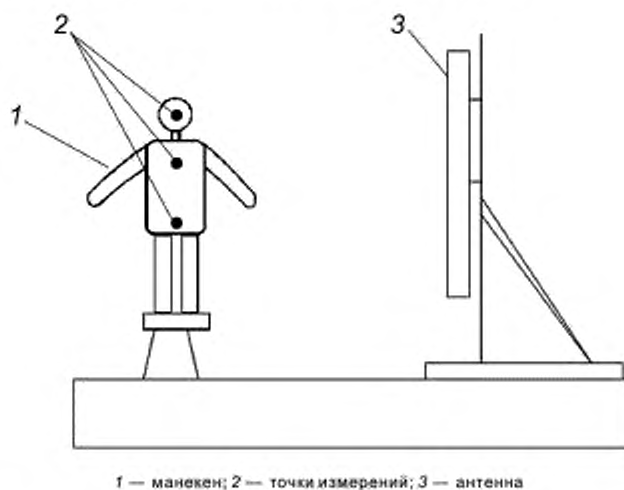
Рисунок 11 — Измерительный стенд для испытаний в свободном пространстве
