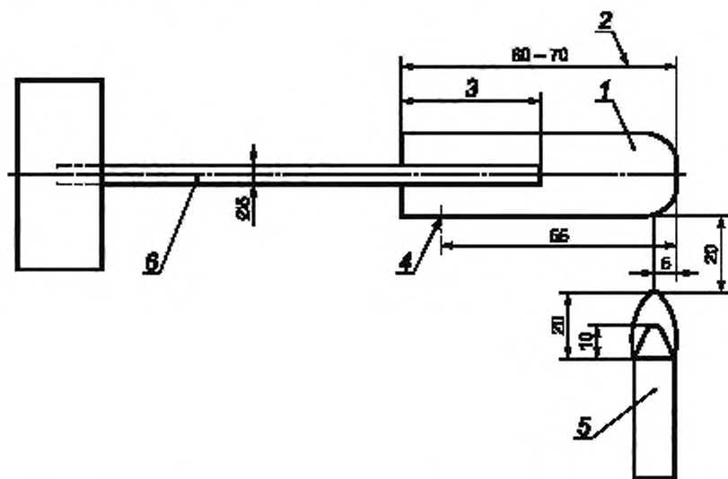
1 — испытуемый образец; 2 — длина испытуемого образца; 3 — половина длины испытуемого образца; 4 — сылочная линия; 5 — горелка; 6 — стальной шпиль
