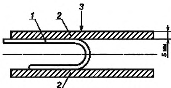
1 — перчатка или рукавица; 2 — полиэтиленовая плита; 3 — прилагаемая сила, равная 100 Н
