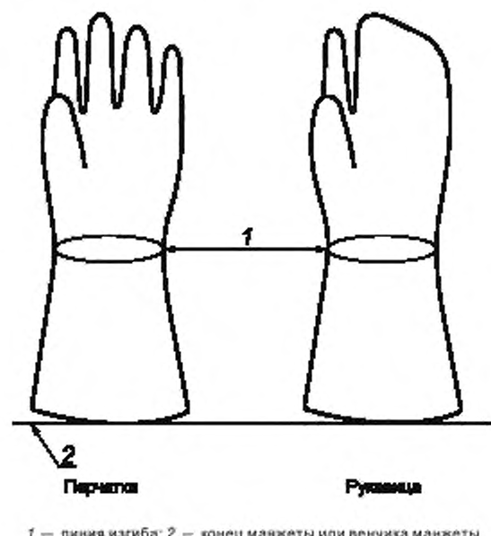
Рисунок 7 — Линия изгиба перчатки при испытании при низких и очень низких температурах
