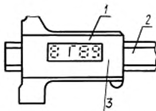
1 — цифровое отсчетное устройство; 2 — штанга; 3 — рамка
