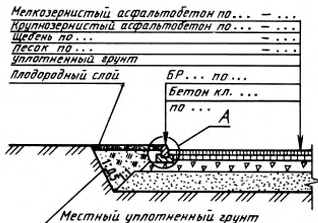
Тротуар (тип 2)
