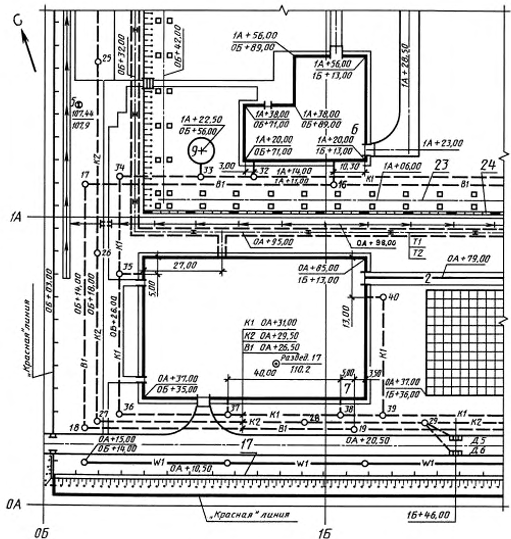
Пример оформления сводного плана инженерных сетей
