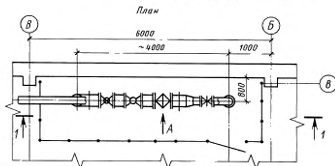
Газорегуляторная установка (ГРУ)
