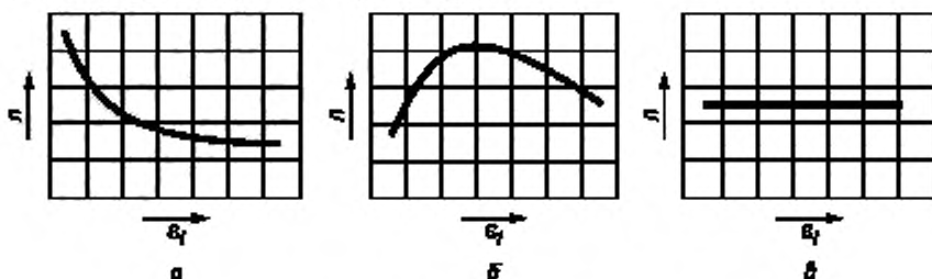
Рисунок Е.1 — Типовые зависимости показателя деформационного упрочнения n от степени деформации \epsilon_j
