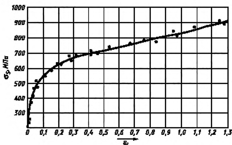
Рисунок 9 — Экспериментальная кривая упрочнения в координатах \sigma_t - \epsilon_t
