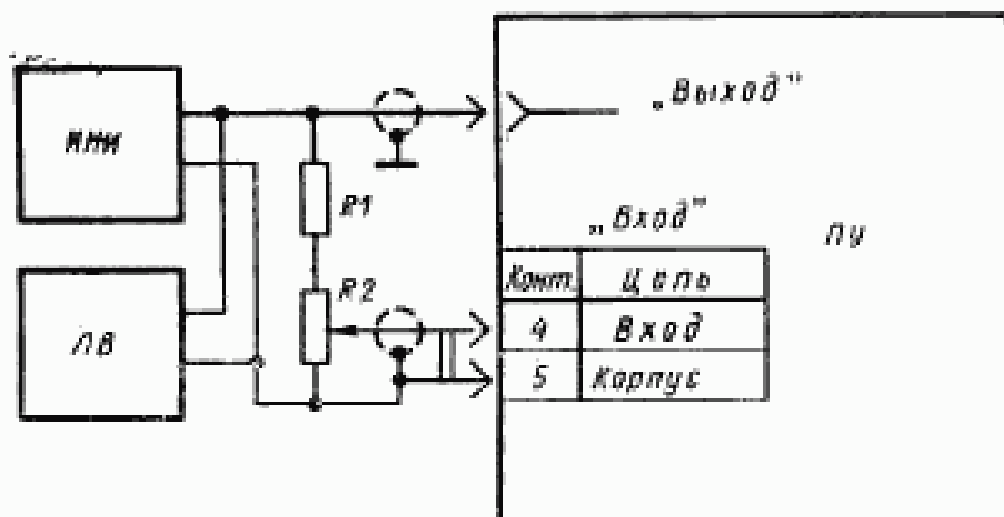
Схема для проверки нелинейных искажений
