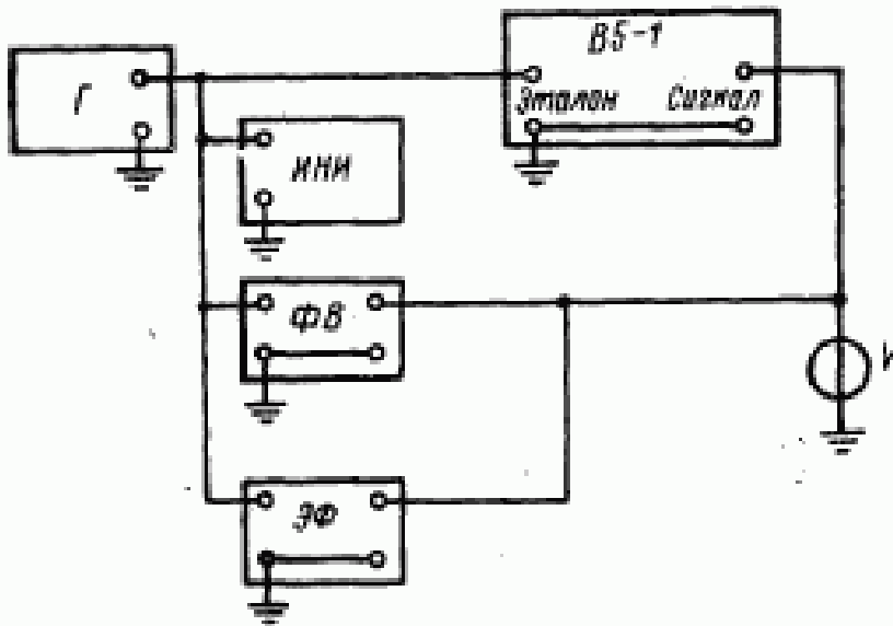
Схема поверки вольтметра В5—1
