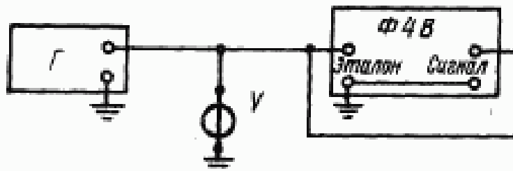
Г—измерительный генератор; V—образцовый вольтметр; ФЧВ—поверяемый фазочувствительный вольтметр.
