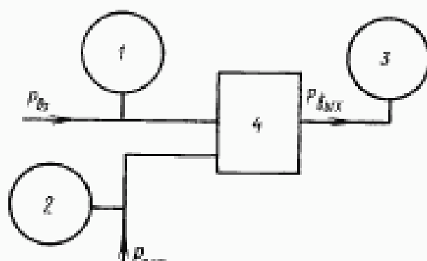
1—образцовый прибор для задания (измерения) входного давления; 2—прибор для контроля давления воздуха питания; 3—образцовый прибор для измерения (заданного) выходного сигнала; 4—поверяемый прибор.
