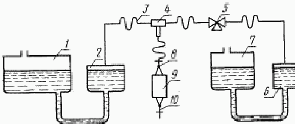
1, 2—подвижный и неподвижный сосуды рабочего эталона; 3—резиновые трубки; 4—тройник; 5—пробковый трехходовой кран; 6, 7—неподвижный и подвижный сосуды поверяемого микроманометра; 8—сифонный пресс с кранами 8, 10
