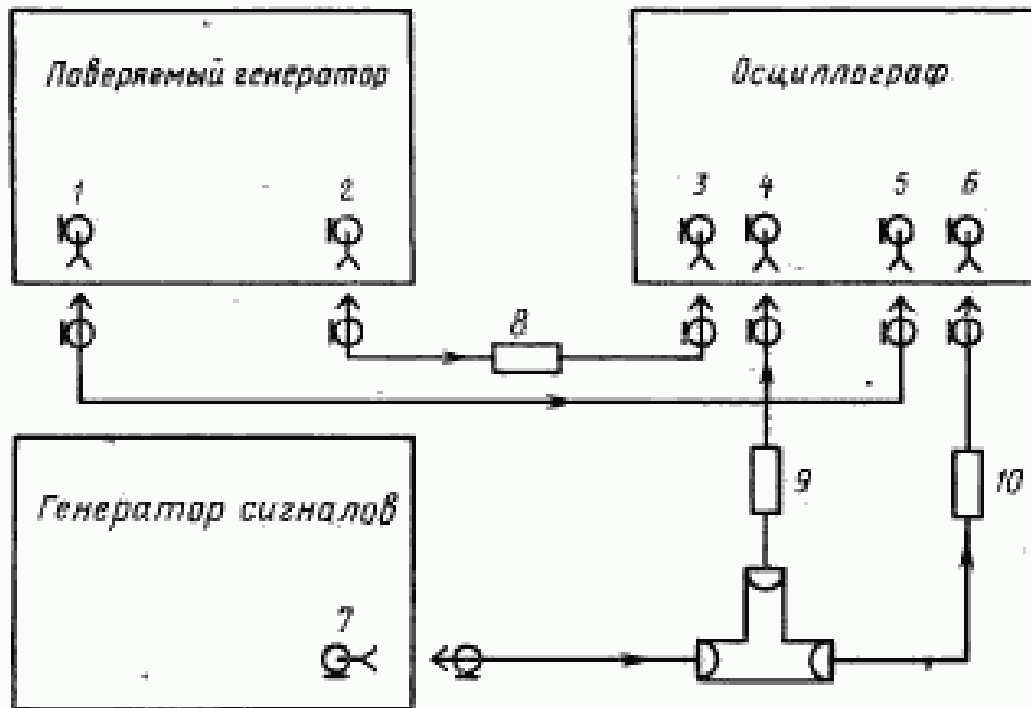
1—выход синхронизирующий импульсов; 2—выход основных импульсов; 3—вход I канала Y; 4—вход II канала Y; 5—вход низкочастотной синхронизации; 6—вход высокочастотной синхронизации; 7—выход сигнала; 8, 9, 10—аттенюаторы
