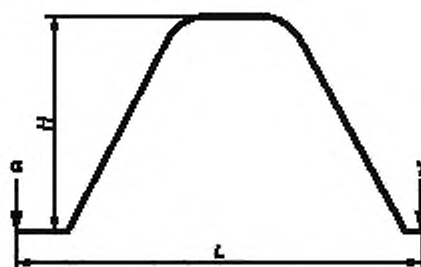
α — точка на видеопрофиле, соответствующая началу положения зонда АСМ при сканировании; γ — точка на видеопрофиле, соответствующая концу положения зонда при сканировании; H — высота выступа, измеренная по видеопрофилю; L — разность абсцисс конечной и начальной точек горизонтального сканирования, соответствующая величине горизонтального перемещения подвижной части рабочего стола АСМ, вычисленная по видеопрофилю
