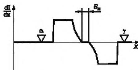
Х — ось абсцисс по 8.2.2; \alpha , \gamma — начальная и конечная точки положения зонда АСМ при сканировании поверяемого элемента, расположенные в соответствии с требованиями по 8.2.1;
