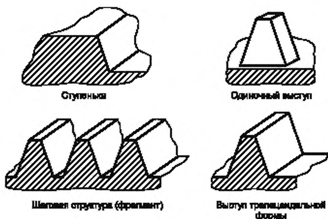
Рисунок 1 — Типовые элементы рельефа рельефной меры
