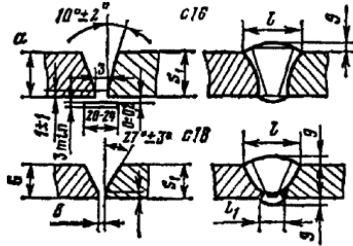
Рис. 2. Конструктивные элементы стыковых швов (а) и последовательность выполнения сварного соединения (б):
