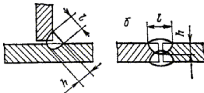
Рис. 9. Типы швов:
