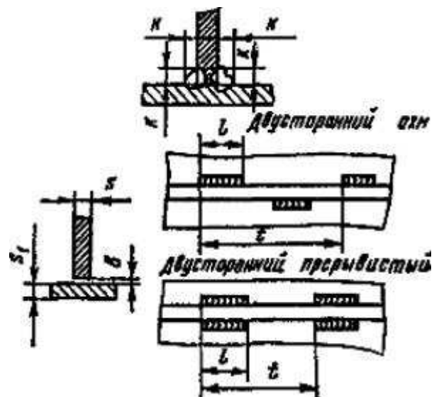
Рис. 4. Сварка угловых тавровых швов:
