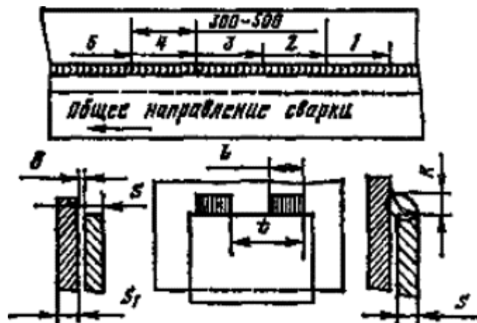
Рис. 3. Сварка нахлесточных швов:
