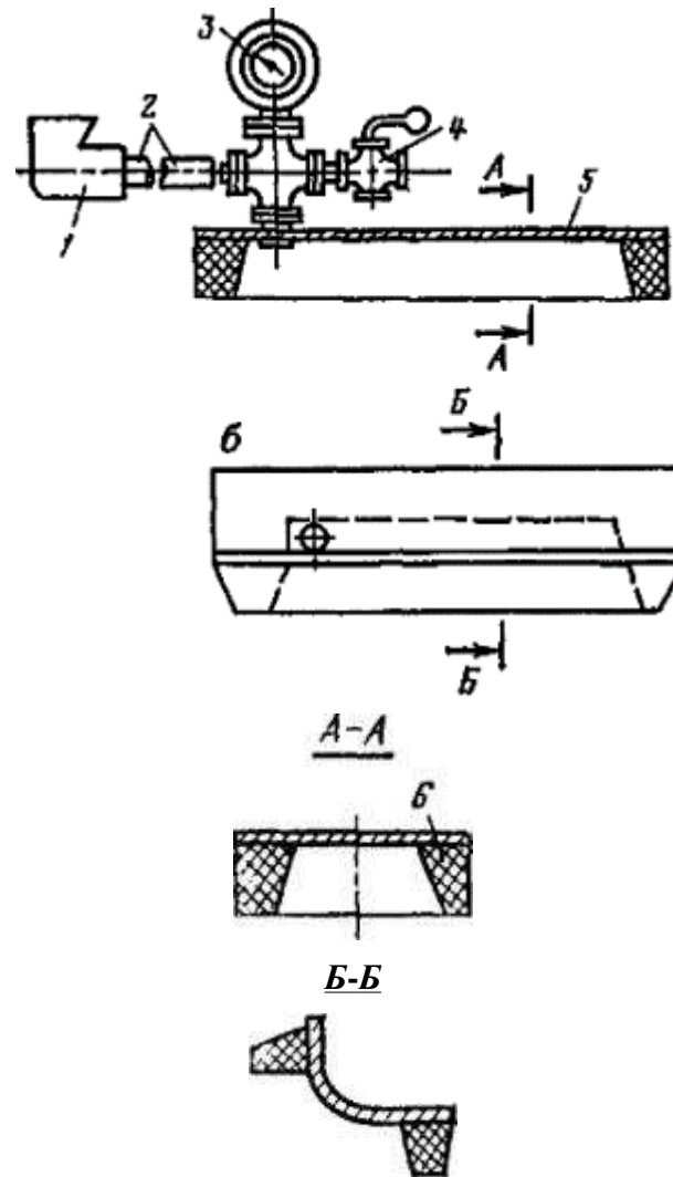
Рис. 5. Вакуумкамеры для испытания герметичности швов:
