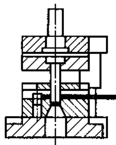
Штамп простого действия для вырубки
