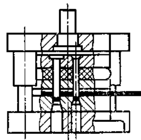
Штамп последовательного действия для пробивки и вырубки
