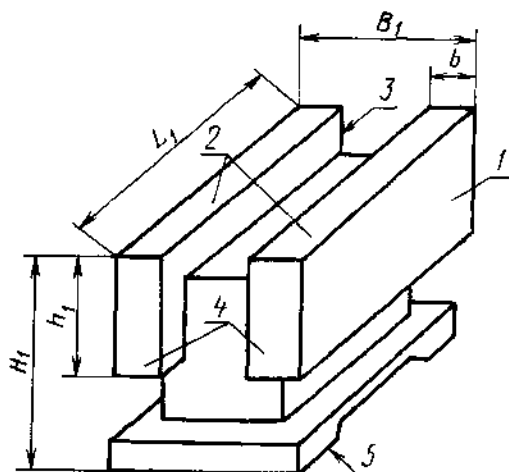
Образец-изделие для станков с горизонтальным фрезерным шпинделем
