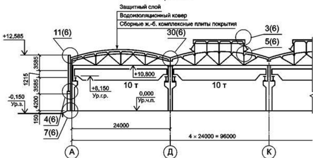
Разрез 1-1
