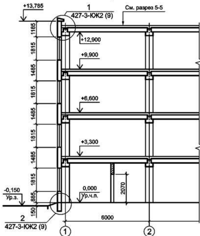
Разрез 2-2
