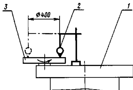
Черт. 10
