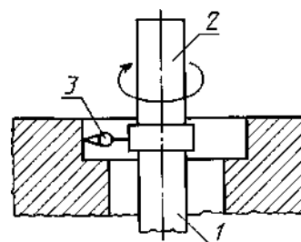
Черт. 10в
