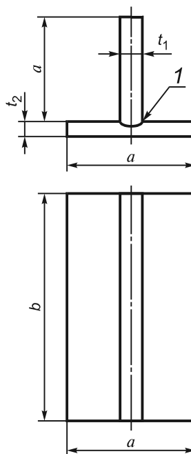
1 — сварной шов с одной или обеих сторон. Подготовка и сборка соединения, как описано в pWPS; a — минимальное значение 150 мм; b — минимальное значение 300 мм; t — толщина материала
