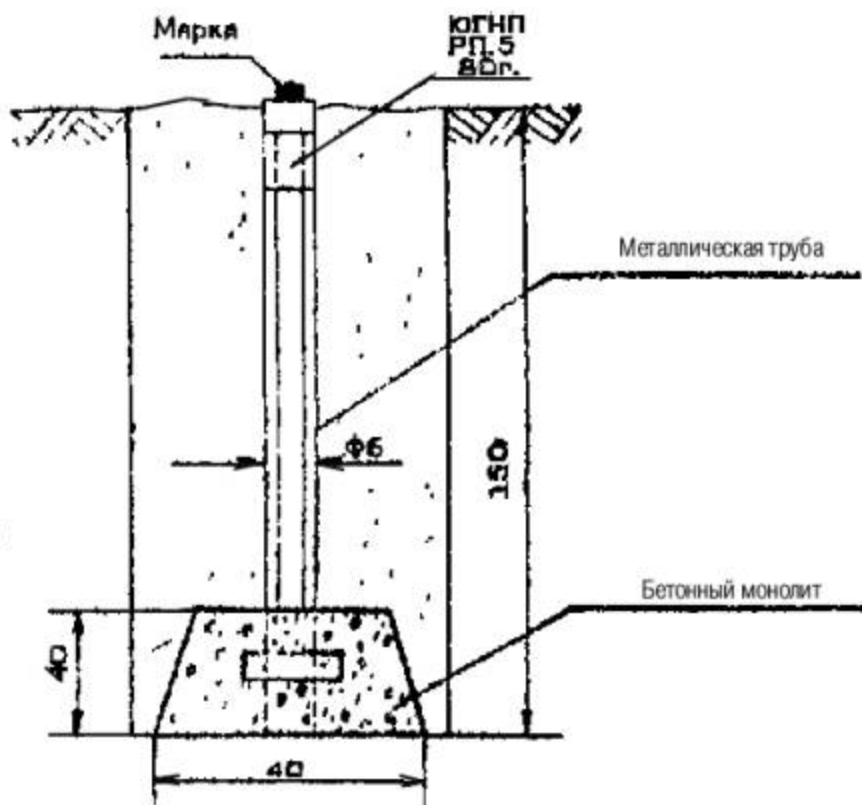
Рис. 12. Тип грунтового репера для открытой местности
