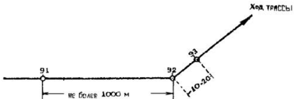
Рис. 1. Закругление угла поворота
