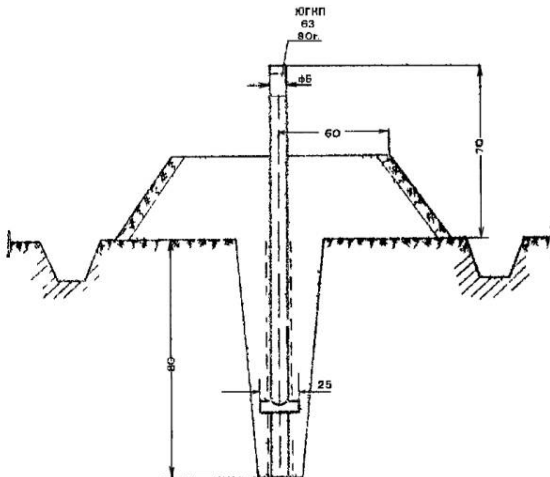
Рис. 5. Тип закрепительного знака с окопкой ровиком
