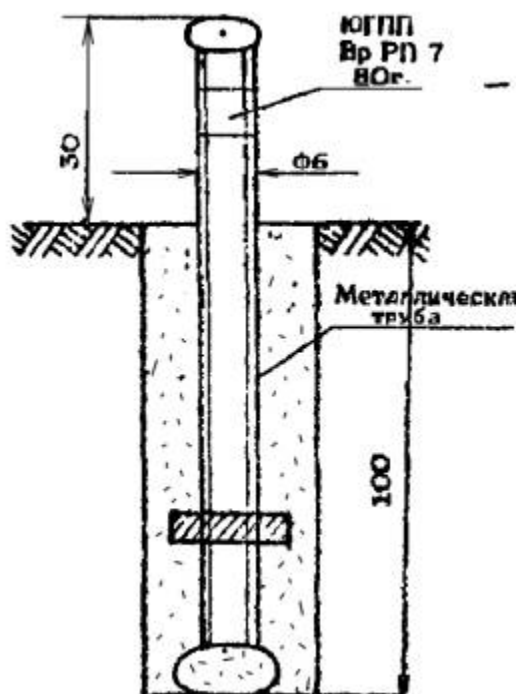
Рис. 7. Тип временного репера заложен в буровую скважину
