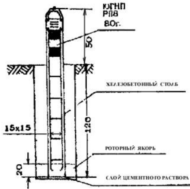
Рис. 14. Тип грунтового репера заложен в буровую скважину
