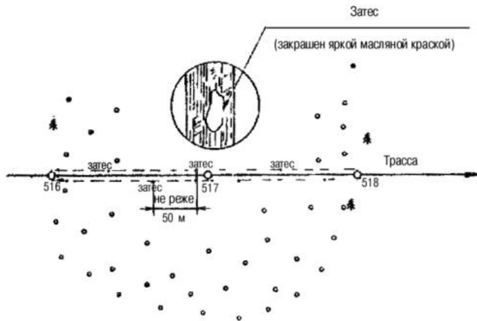
Рис. 3. Закрепление трассы, проходящей через лес
