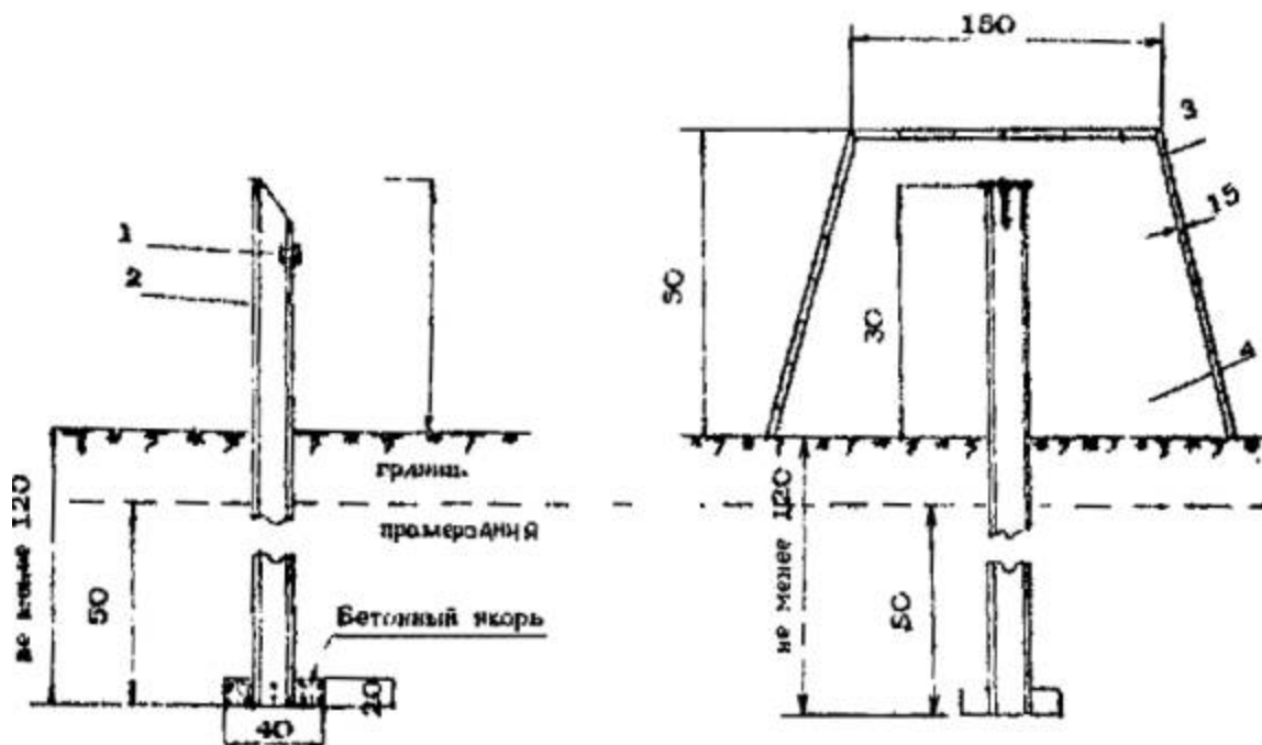
Рис. 10. Тип грунтового репера (размеры в см)
