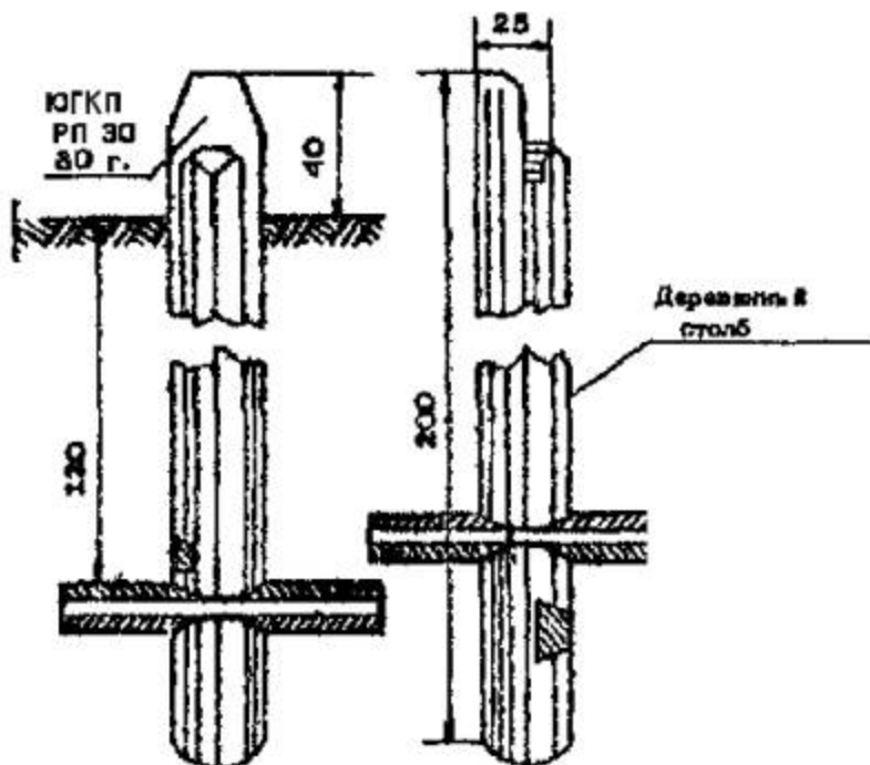
Рис. 6. Тип закрепительного знака (временный репер)
