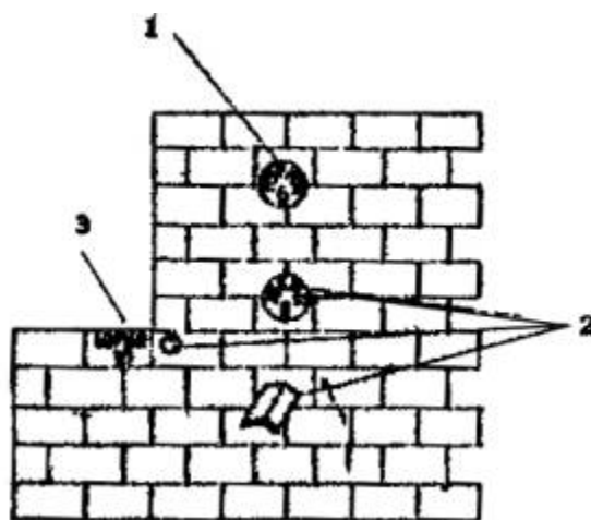
Рис. 9. Стенные реперы
