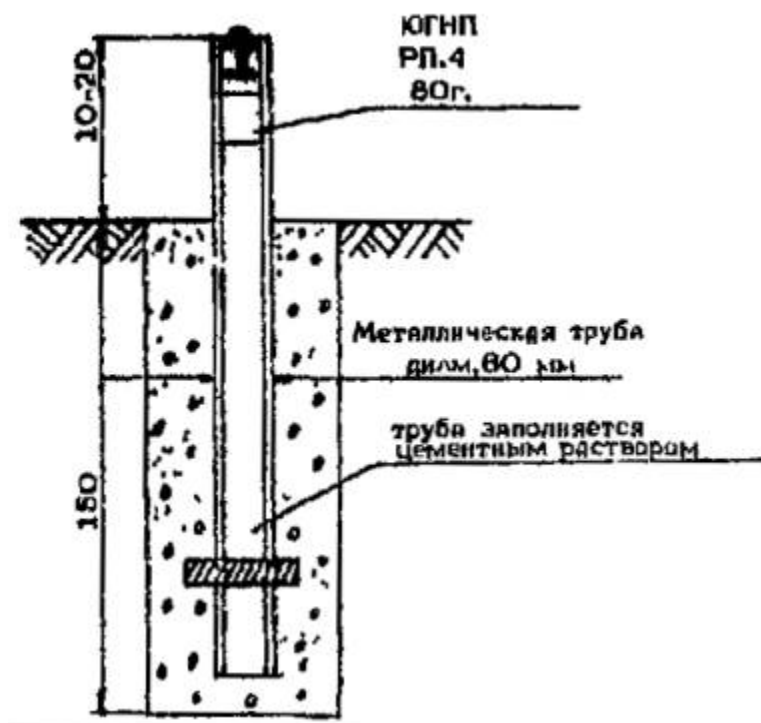
Рис. 12. Тип грунтового репера для открытой местности
