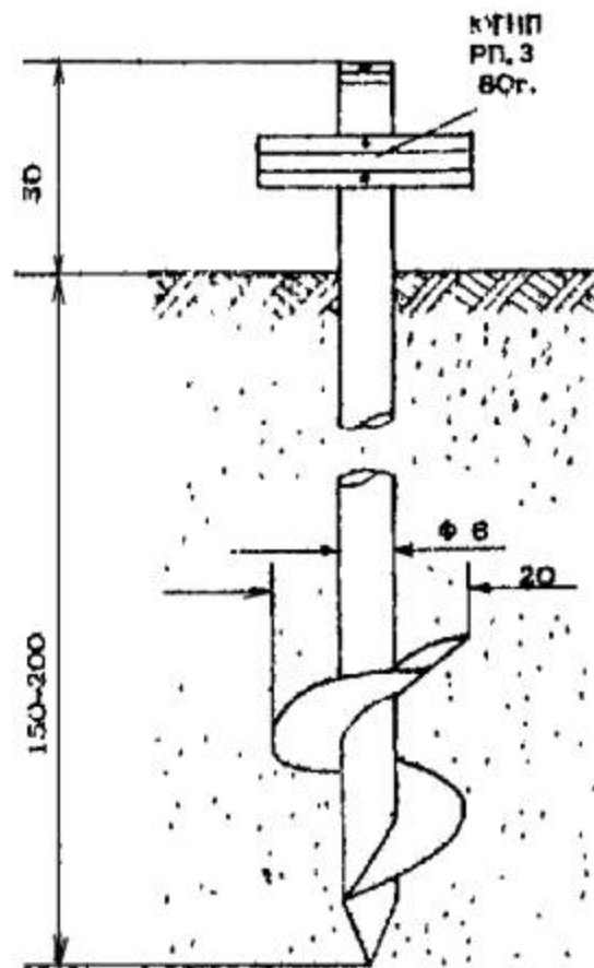
Рис. 11. Грунтовый репер для районов подвижных песков и торфяников
