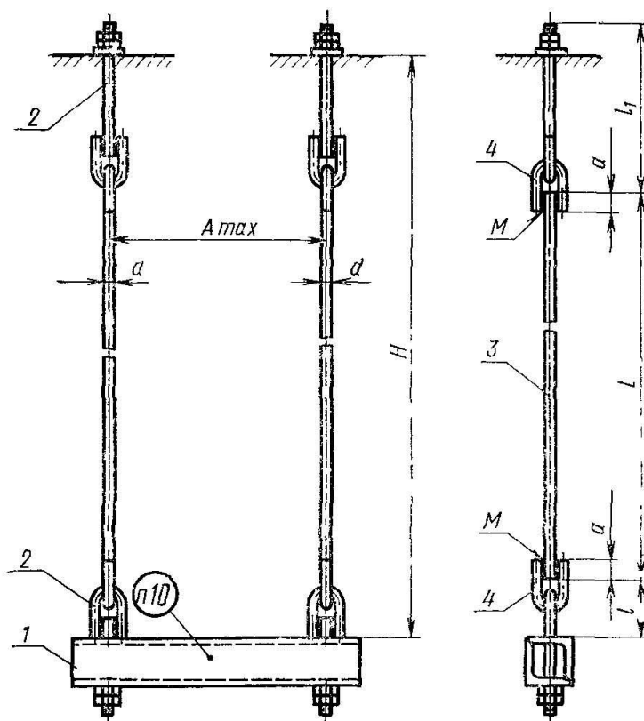
1—балка; 2—тяга большая с ушком; 3—тяга; 4—ушко.
